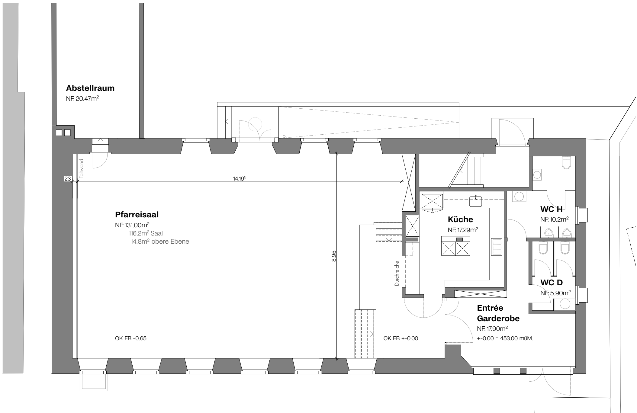
Grundriss Erdgeschoss
